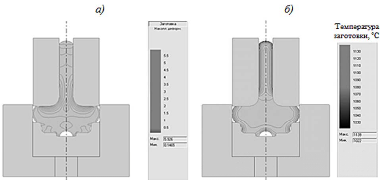
Рисунок 1. Распределение накопленной деформации (а) и температуры (б) в виде изолиний
