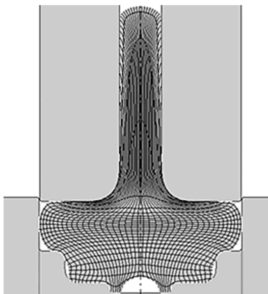
Рисунок 2. Распределение лагранжевых линий в заготовке
